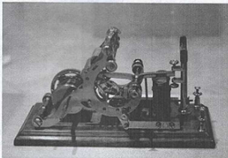
Primer telégrafo receptor automático de señales (1837).
